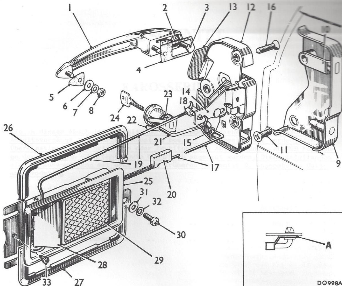
Abb. R.11 Montagebild des Türschloßmechan.
